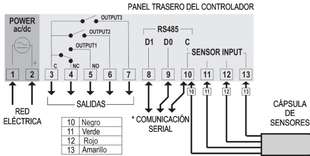
Figura 2 – Terminales del N323RHT – Modelo Patrón
