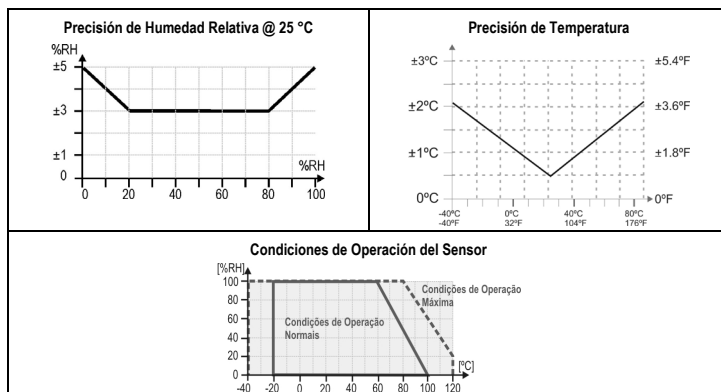
Figura 1 - Precisión en la medición de humedad y temperatura
