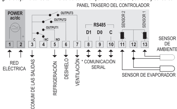
Fig. 1 – Conexiones mostradas en la etiqueta del controlador
