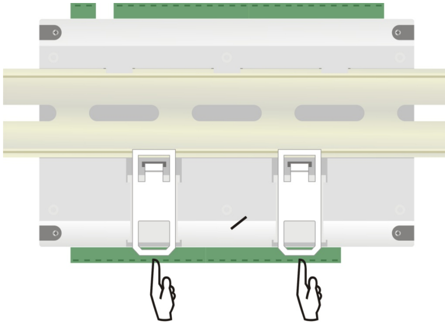
Fig. 03 - Modo de instalación en carril DIN
