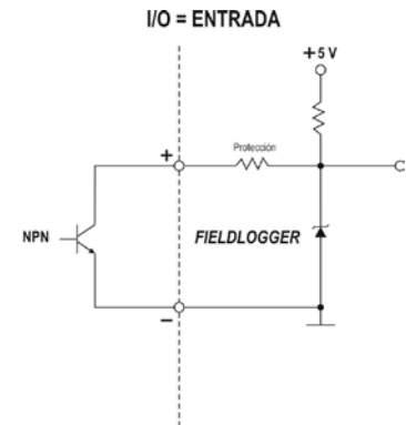
Fig. 17 - Conexión NPN
