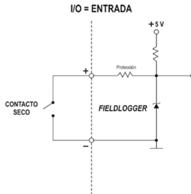
Fig. 16 - Conexión contacto seco
