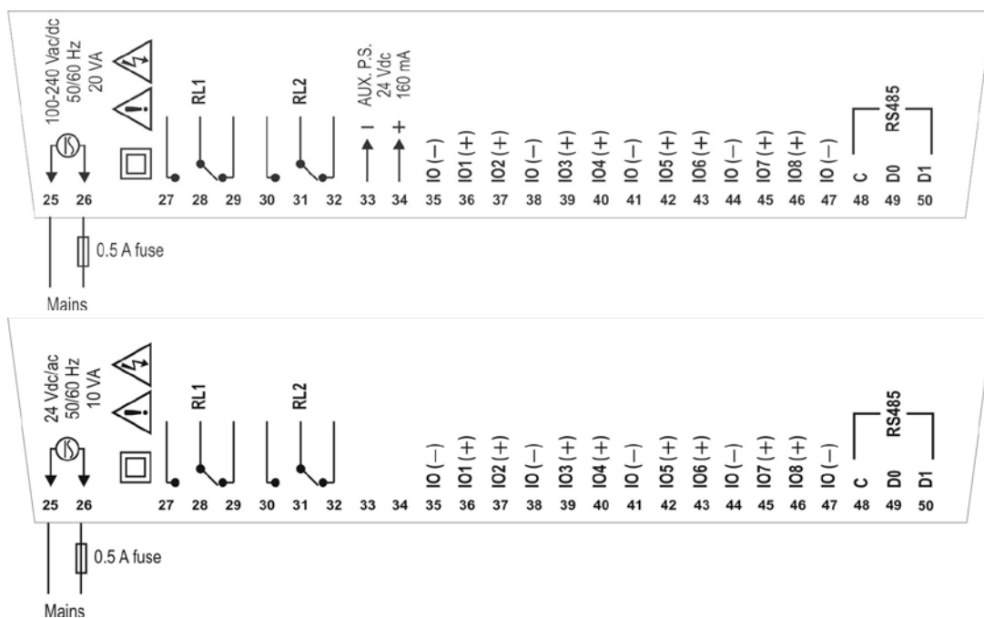
Fig. 13 – Conexiones del lado superior para la versión estándar e 24V
