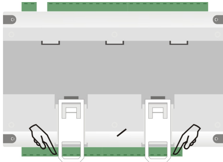
Fig. 01 – Modo de instalación en carril DIN
