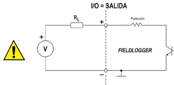
Fig. 18 - Conexión de una carga a la salida digital
