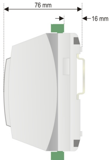
Fig. 07 – Dimensiones del lateral del FieldLogger con módulo IHM
