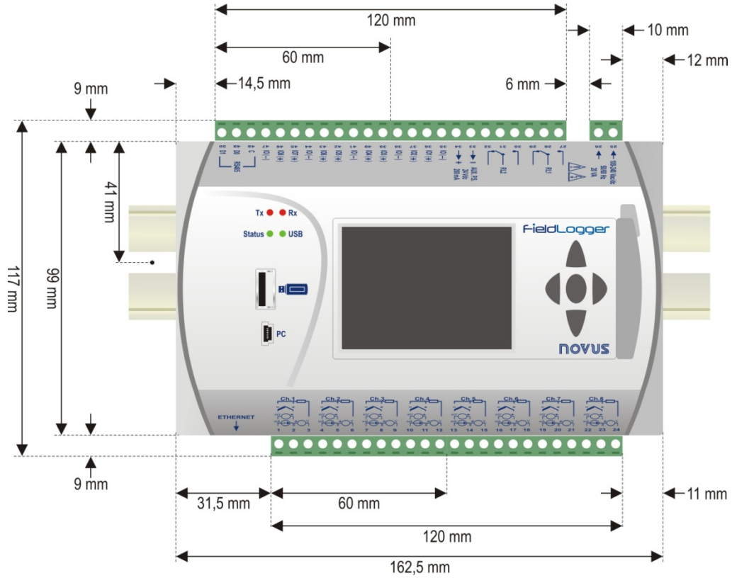
Fig. 06 – Dimensiones del FieldLogger con módulo IHM
