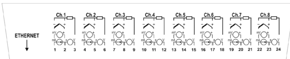
Fig. 14 – Conexiones lado inferior
