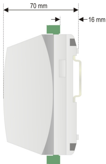
Fig. 05 – Dimensiones del lateral del FieldLogger sin módulo IHM
