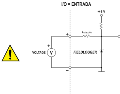
Fig. 15 - Conexión de tensión
