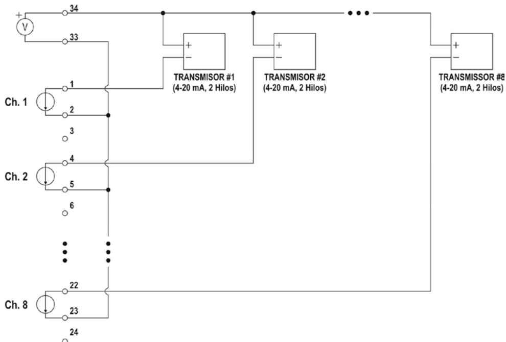
Fig. 19 – Fuente auxiliar para alimentación de transmisores 4-20 mA (2 hilos)
