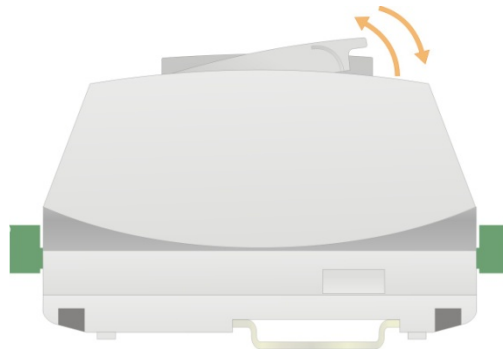
Fig. 11 – Removiendo e instalando la IHM en el FieldLogger (vista lateral)
