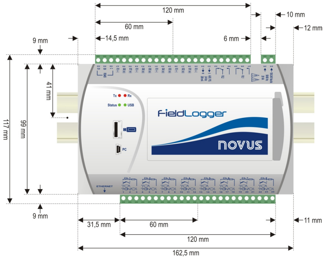
Fig. 04 – Dimensiones del FieldLogger sin módulo IHM
