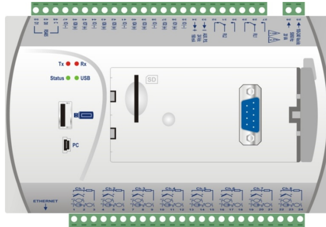
Fig. 20 – Recursos de conectividad del FieldLogger
