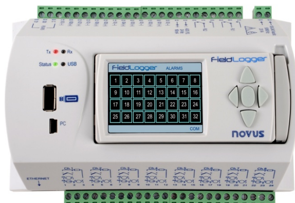
Fig. 25 – FieldLogger con IHM
