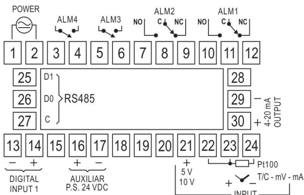
Fig. 1 - Conexiones del panel posterior
