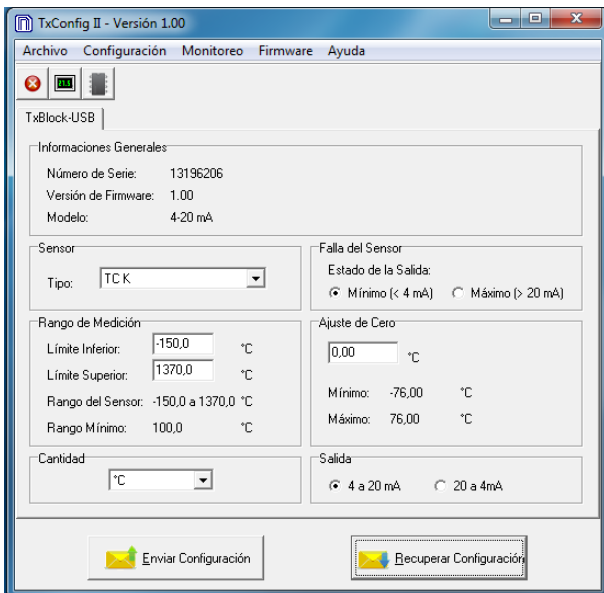
Fig. 10 – Pantalla principal del software TxConfig II
