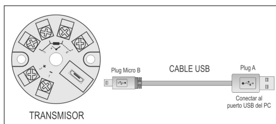
Fig. 8 – Conexión del cable USB
