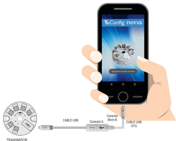
Fig. 12 – Conexión del cable On the Go
